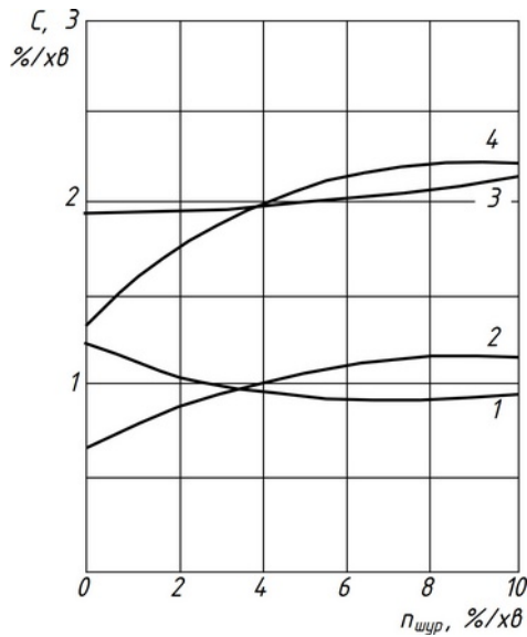
Рис. 3. Залежність швидкості горіння зольного палива від інтенсивності шурування шару: вугілля із зольністю A^p = 14,3 \% : 1 – протягом дослідів; 3 – за період інтенсивного горіння; вугілля із зольністю A^p = 25,5 \% : 2 – протягом дослідів; 4 – за період інтенсивного горіння
