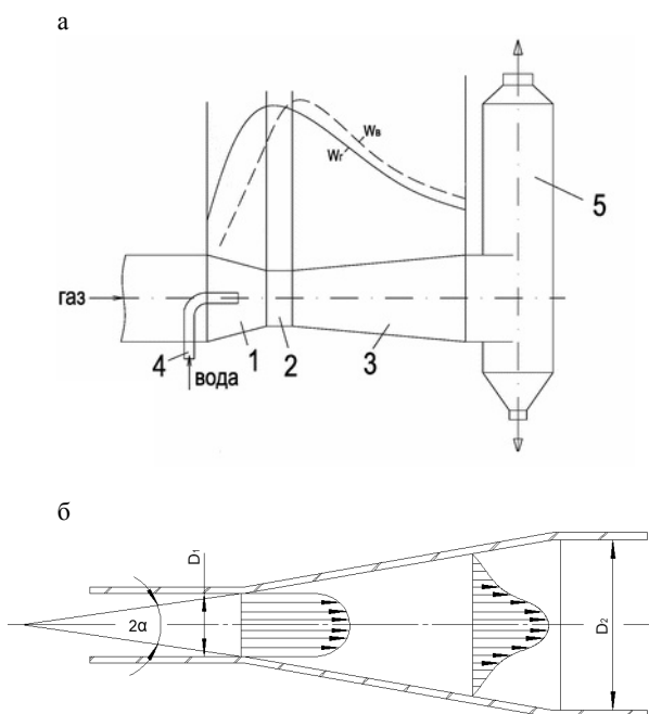
Рис.1 . Скрубєр з трубою Вентурі: а – принципова схема; б – зміна профілю швидкостей за довжиною труби: 1 – конфузор; 2 – горловина; 3 – дифузор; 4 – форсунка; 5 – краплевловлювач; W_l – зміна швидкості рідини, м/с; W_g – зміна швидкості газу, м/с
