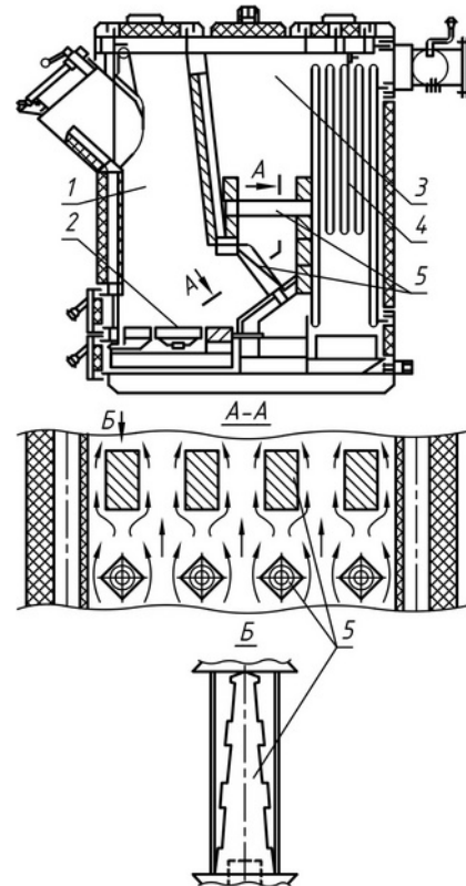
Рис. 4. Котел для спалювання дерев, кускового торфу та відходів деревини 1 – паливна шахта; 2 – решітка; 3 – камера згорання; 4 – конвективні поверхні; 5 – змішувач газоповітряної суміші
